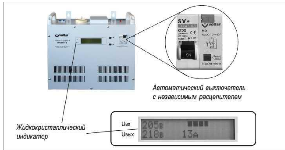
Фіг. 2. Стабілізатор лицьової пластини
