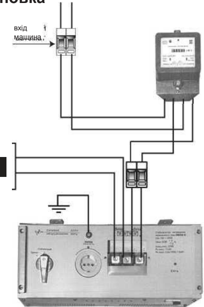
Фіг. 10. Схема установки стабілізатора
