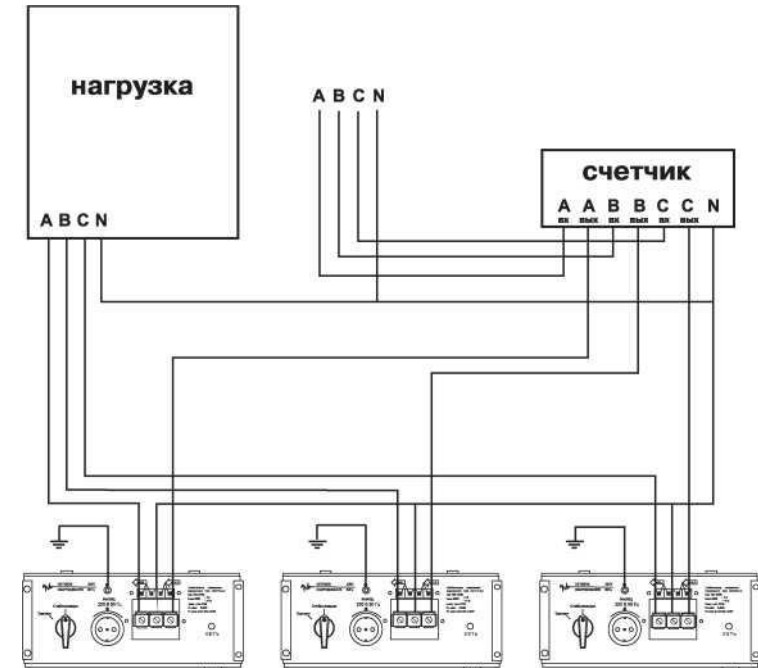
Фіг. 18. Схема підключення стабілізаторів до трифазної мережі
