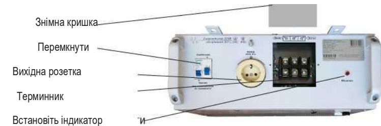
Фіг. 4. Верхня панель стабілізатора
