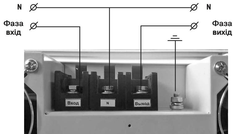
Мал.4. Схема підключення стабілізатора
