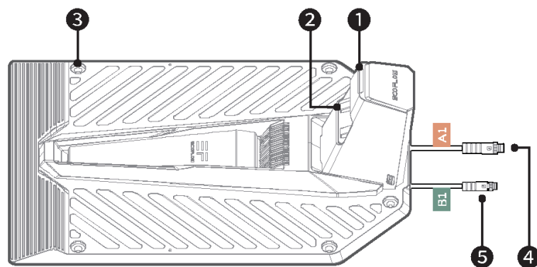
Рис. 4 Зарядна станція
