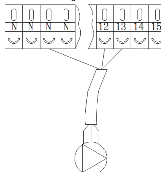
1# elektromagnetisches Drei-Wege-Ventil
