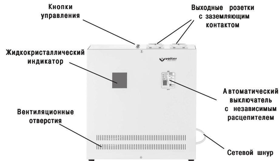
Рис. 1. Стабилизатор напряжения Etalon-2.
