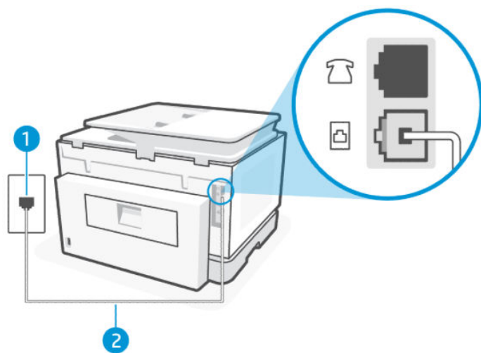
Таблиця 7-4 Вигляд принтера ззаду
