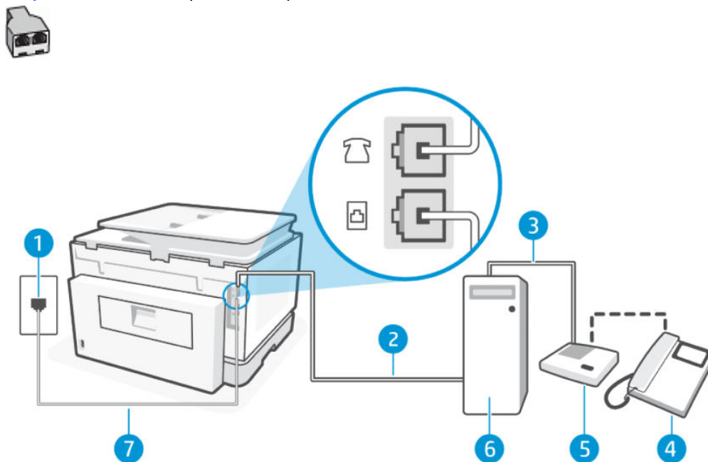
Рисунок 7-4 Вигляд паралельного розділювача
