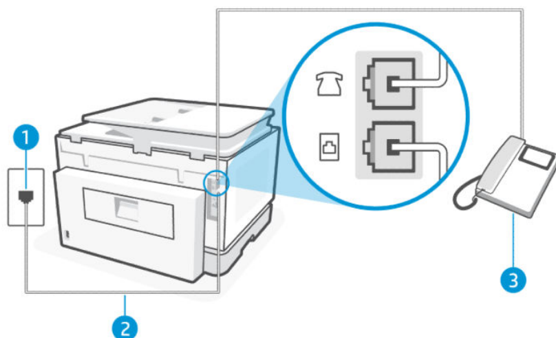
Таблиця 7-7 Вигляд принтера ззаду
