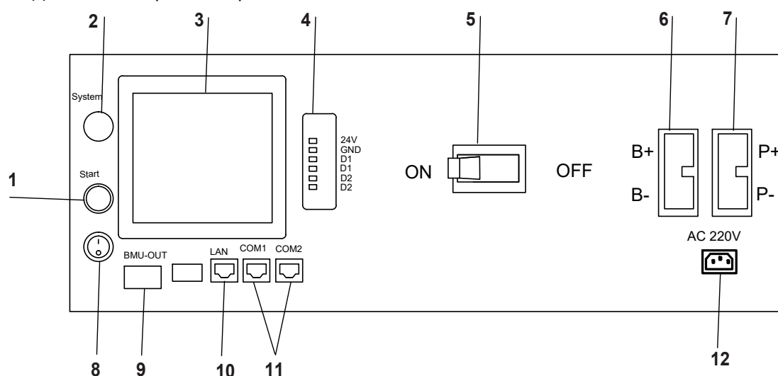
зовнішній вигляд BMS 125A
