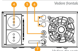
Vedere din spate pentru Aira 600
