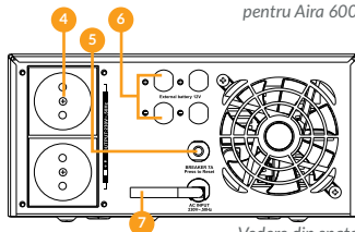
Vedere din spate pentru Aira 1200
