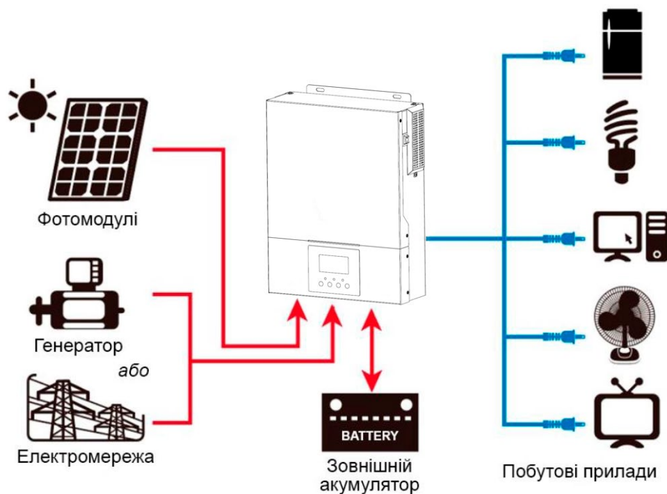
Зображення 1. Гібридна система живлення
